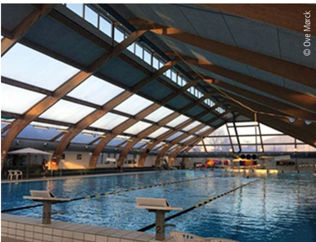
Die Schwimmhalle vor der Sanierung mit dem aufgeblasenen Kunststoffdach auf der Dachkonstruktion
