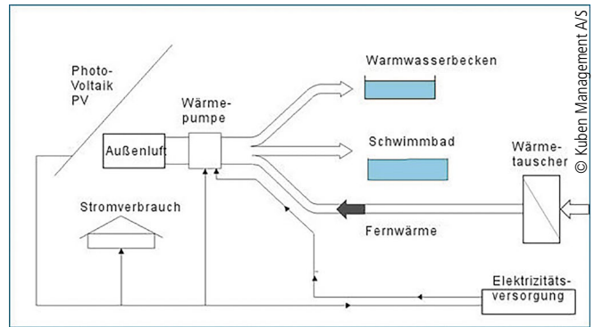
Das Funktionsprinzip des Energiesystems der sanierten Schwimmhalle. Den erneuerbaren PV-Strom leiten die Betreiber entweder in die Schwimmhalle oder zur Wärmepumpe.
